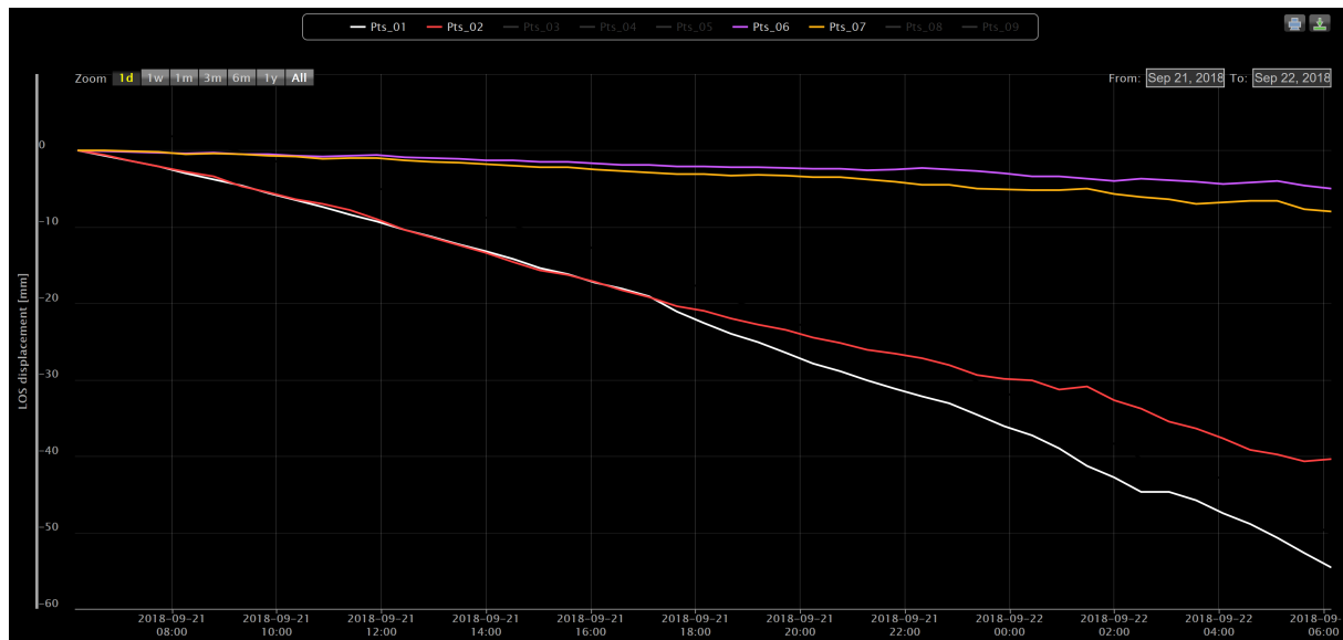
Figur 1: Bevegelse på radarpunkter siste døgn i øvre del (P1 og P2) og nedre del (P6 og P7)
